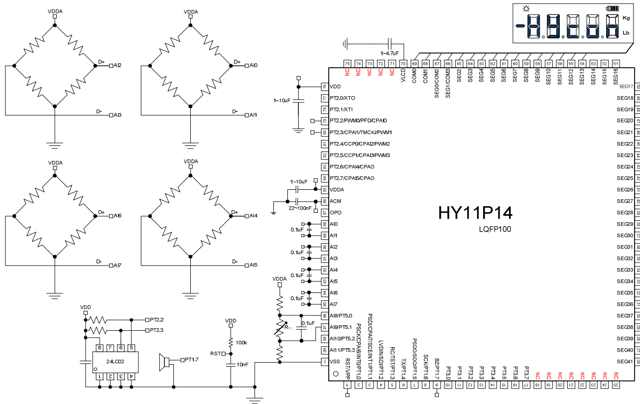
圖 3-1 具溫度補償的橋式感測器應用電路
