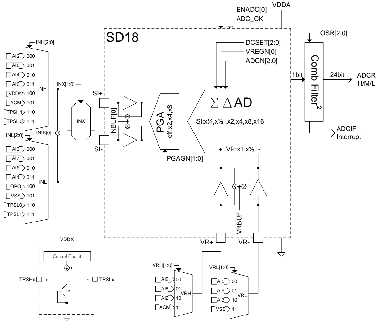
圖 4-2 SD18 Network
