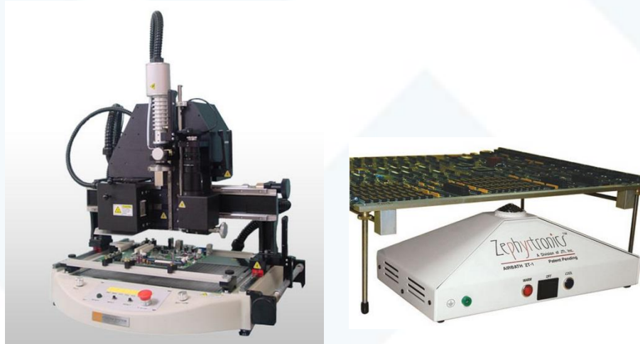
圖十 常見的預熱機 / 預熱板
