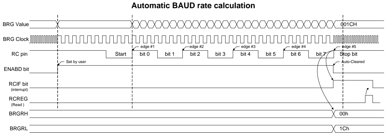
圖 14-1 自動鮑率計算波形
