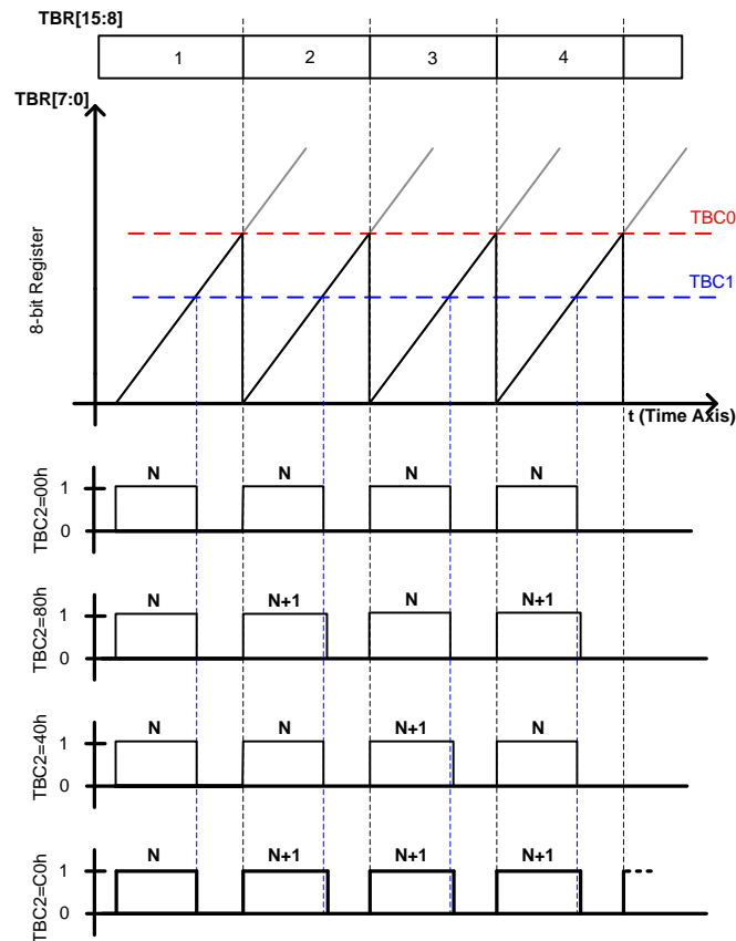
圖 10-10 PWM50 輸出波形示意圖 1
