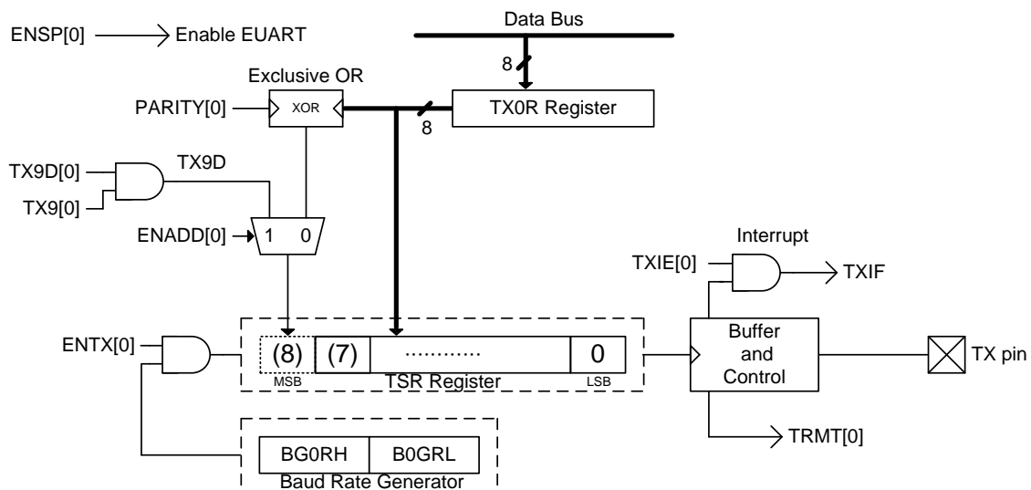
圖 14-3 EUART 傳送方塊圖
