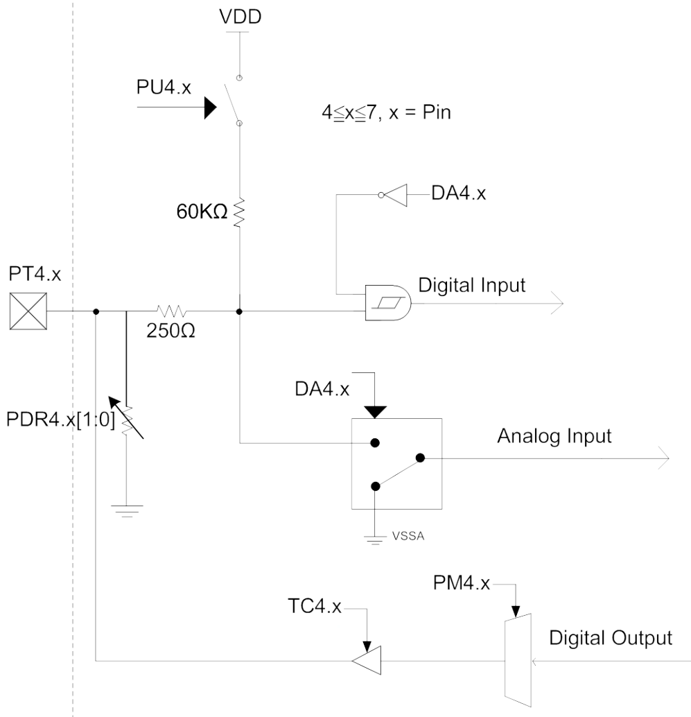
圖 7-2PT4.x I/O 架構方塊圖
