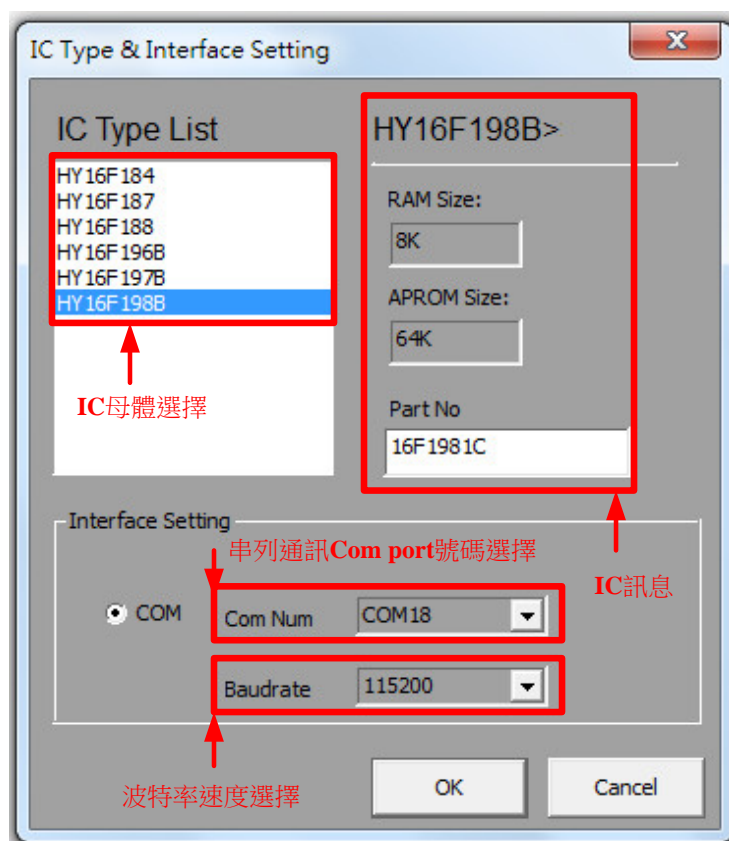
圖 4. IC 母體選擇對話方塊
