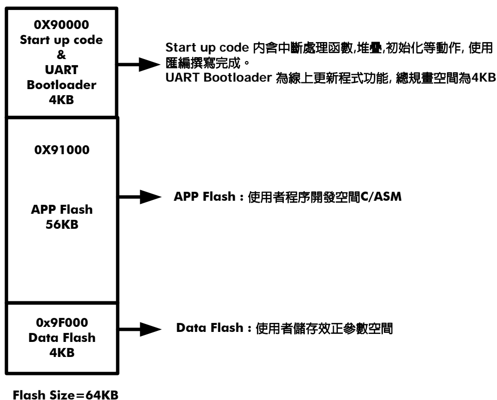
Flash 功能區塊分佈
