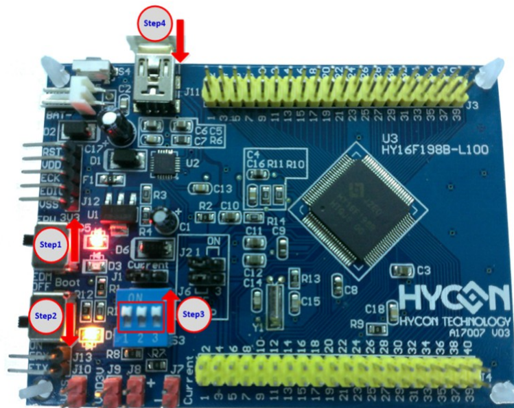
圖 9. 硬體實物連接圖
