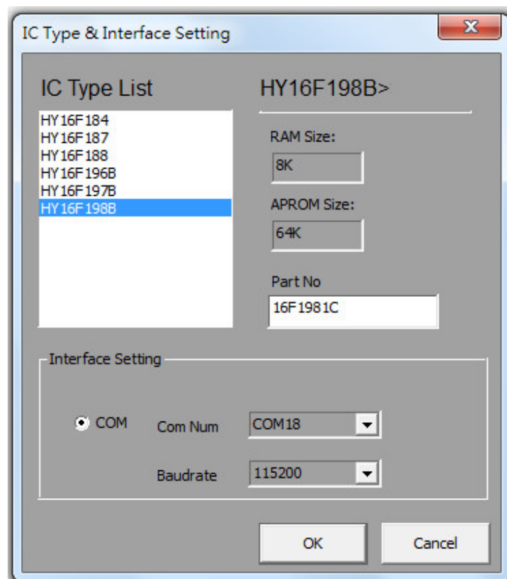
圖 1. IC 選型畫面
