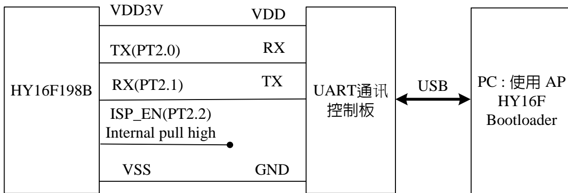
圖 8. 系統連接架構圖
